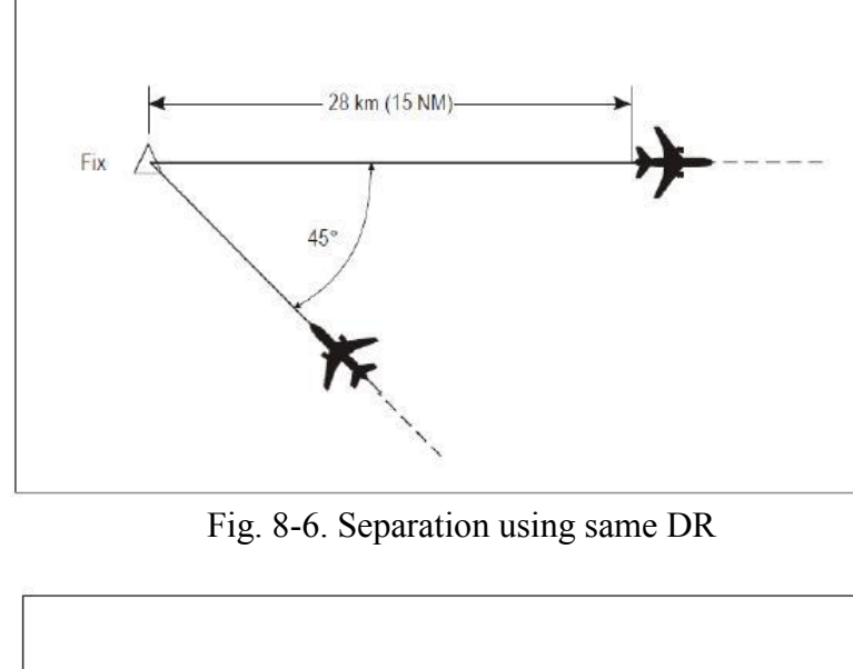
Fig. 8-6. Separation using same DR
