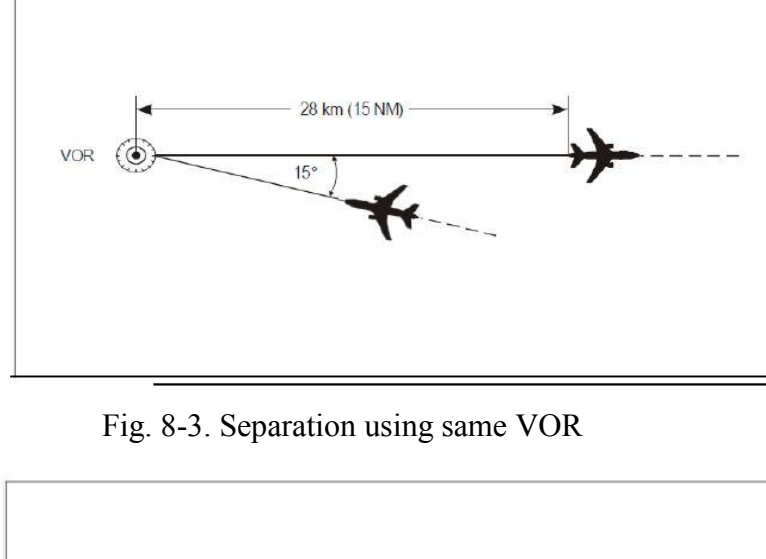
Fig. 8-3. Separation using same VOR
